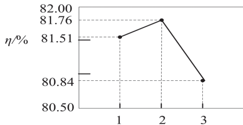
(a) B_{s2} 与效率 \eta 的对应关系
