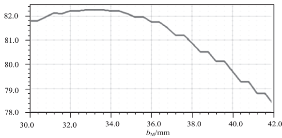
图 4 永磁体宽度与效率关系
