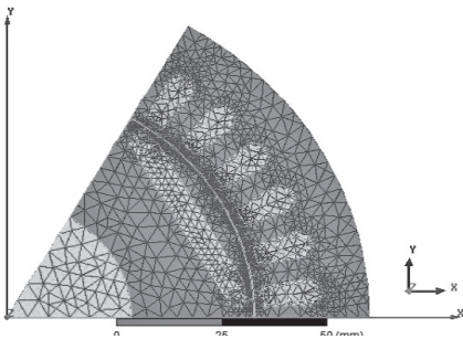
图 8 网格剖分
