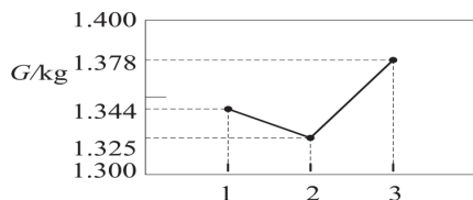
(b) B_{s2} 与永磁体重量 G 的对应关系
