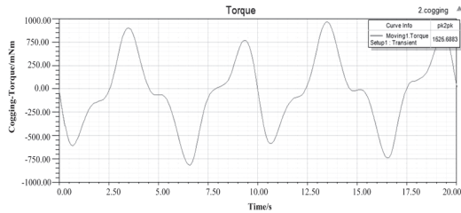
图 11 齿槽转矩波形
