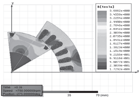
(a) 磁力线
