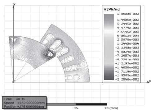
(b) 磁密分布
