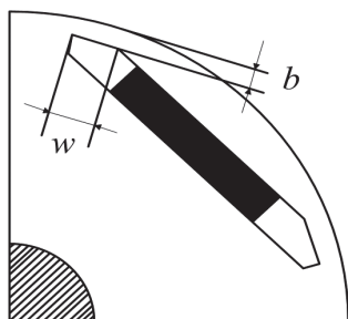
图 5 IPMSPM 隔磁桥
