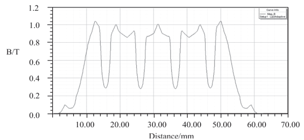
图 10 气隙径向磁密波形
