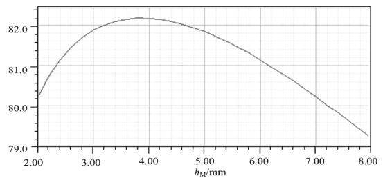
图 3 磁化方向厚度 h_M 与效率关系
