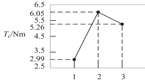
(c) B_{s2} 与齿槽转矩峰峰值 T_c 的对应关系
