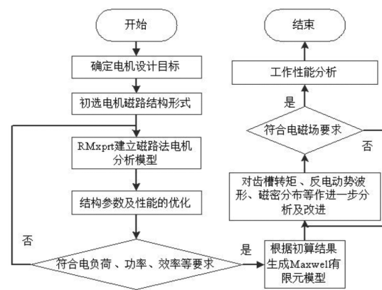
图 1 IPMSPM 设计流程
