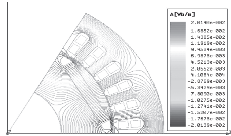
(a) 磁力线
