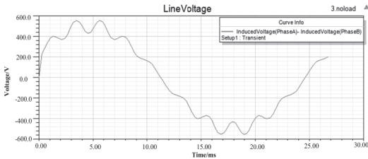
图 12 线电压空载反电势波形
