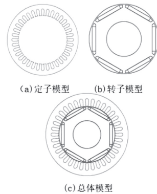
图 2 IPMSPM 的 RMxpert 模型
