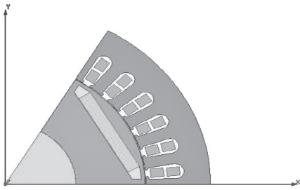
图 7 Maxwell 2D 模型
